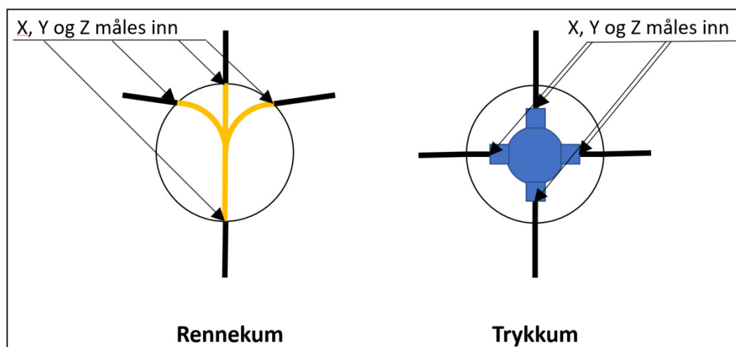
Figur 7 Hvordan måle inn ledning ved kum.
