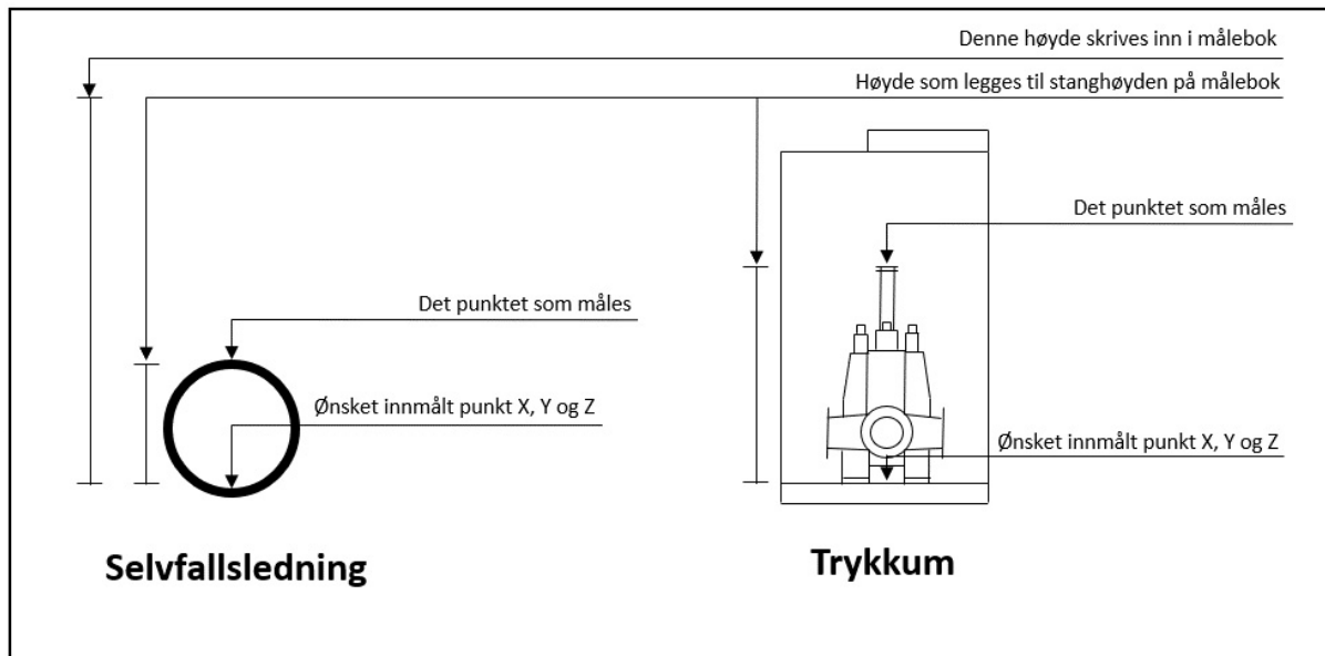
Figur 9 Eksempel innmåling punkt som ikke er synlig.
